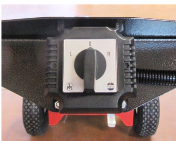
Bouton Marche/Arrêt avec sens de rotation sur balayeuse radiale FKE 800
